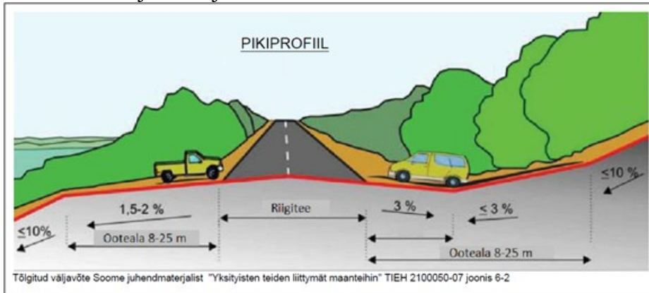
Joonis 2. Ristumiskoha pikikaldete kujundamine
